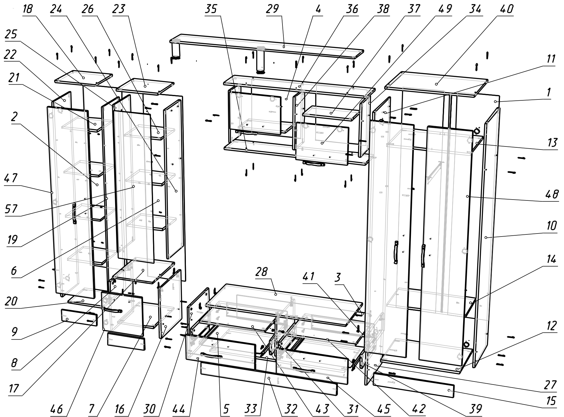
Схема сборки. Гостиная Оскар
